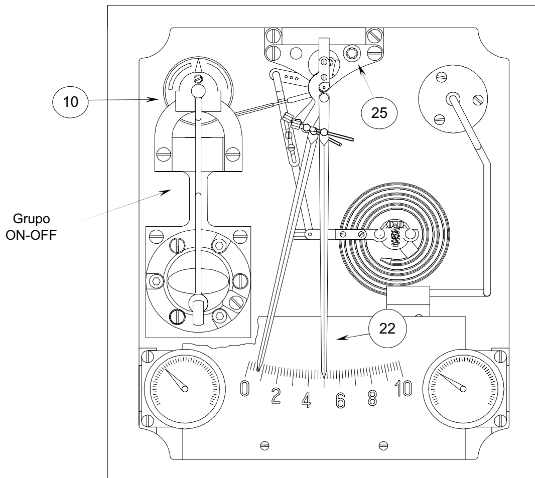
Fig. 3.1.1 "REGULADOR SERIE 350 ON-OFF" (presión)
