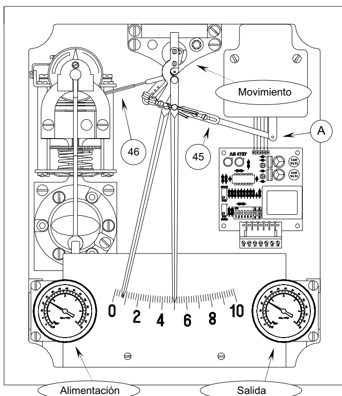
Fig. 8.2.1 "REGULADOR SERIE 700EP"
