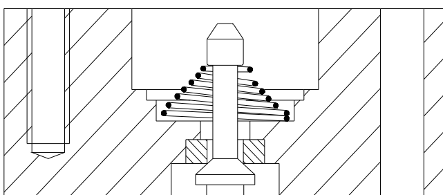
Fig. 6.3.4 "ASSEMBLAGE DES ELEMENTS (38), (39) ET (41)"
