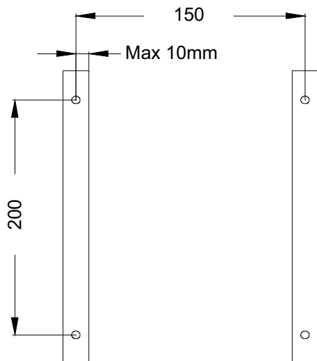
Fig. 1.2.1 "ENTRE-AXES MONTANTS"
