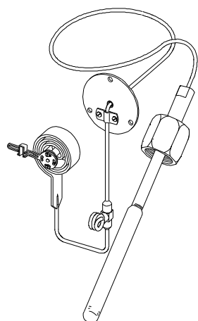
Elément de température complet
