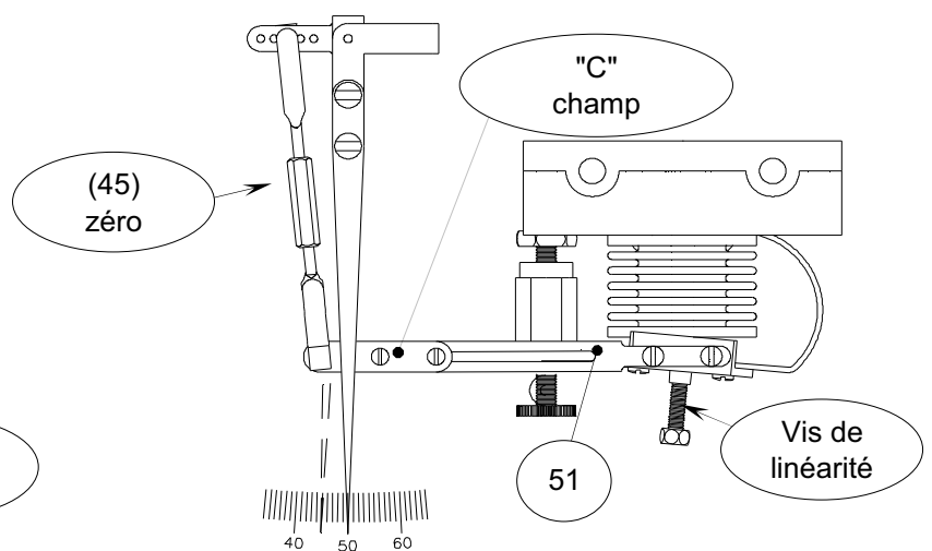
Fig. 8.1.2 "ELEMENT RECEPTEUR 3÷15 psi"
