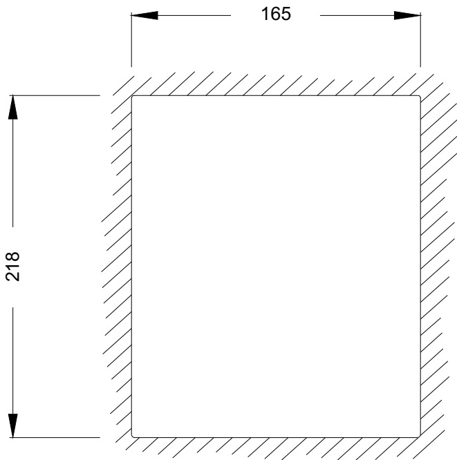
Fig. 1.1.1 "PERCAGE PANNEAU"
