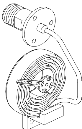
Elément de pression complet
