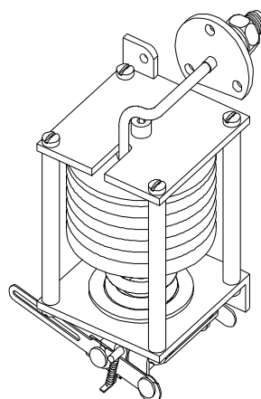
Elément de basse pression complet
