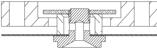
Fig. 14.3.3 "MONTAJE ELEMENTOS (32) Y (35)"
