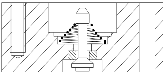
Fig. 14.3.4 "MONTAJE ELEMENTOS (38), (39) Y (41)"
